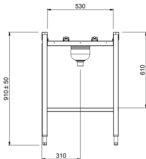
Zij aanzicht
