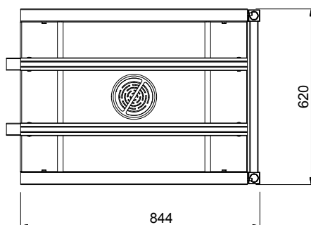
Boven aanzicht
